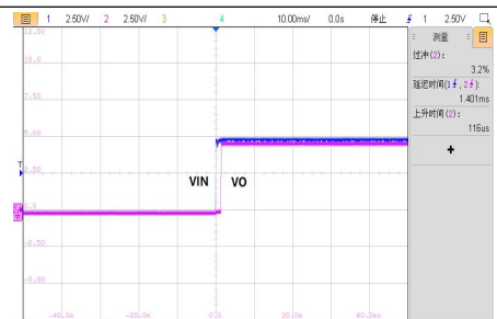
VIN=5.0V, 满载启机波形
