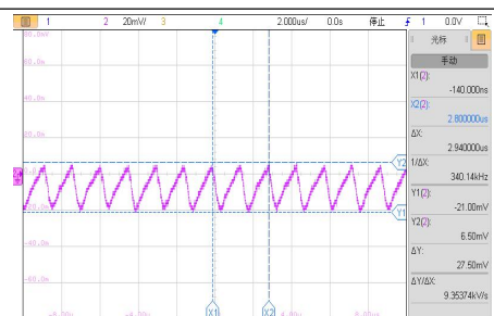
VIN=5.0V, 满载输出电压纹波波形
