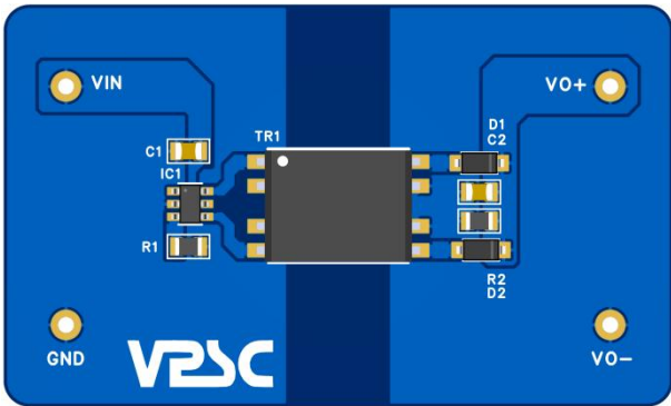
图 1: VPS8702B Demo 板 (50mm*30mm)
