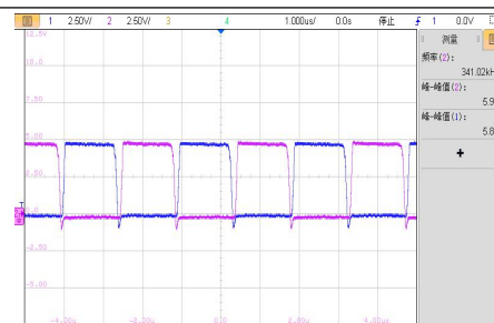
VIN=5.0V, 半载 VDS 波形
