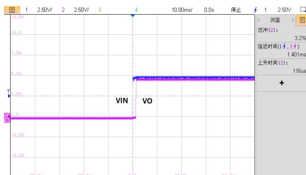
图 4: VIN=5V, IO=200mA,VO 启机波形
