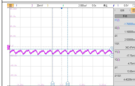
VIN=5V, 轻载输出电压纹波波形
