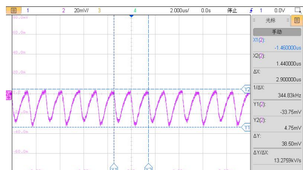
图 5: VIN=5V, IO=200mA,VO 输出电压纹波波形
