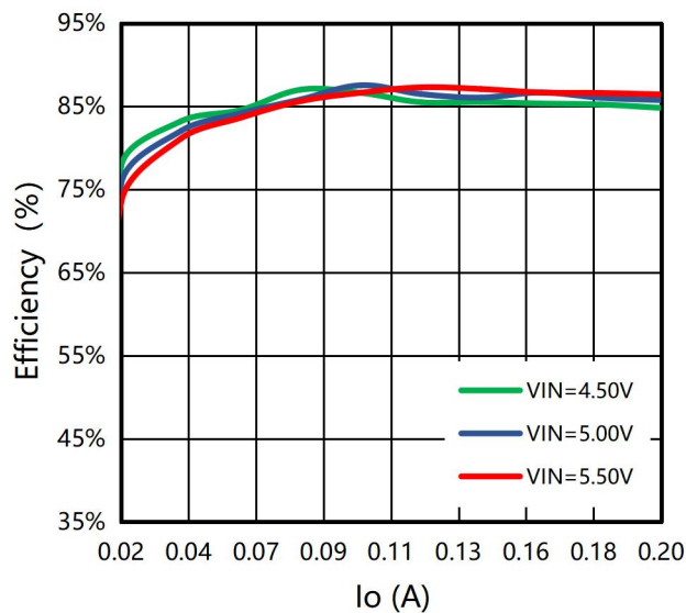
图 2: IO=0-200mA,效率 VS 输出电流
