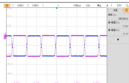
VIN=5V, 满载工作波形
