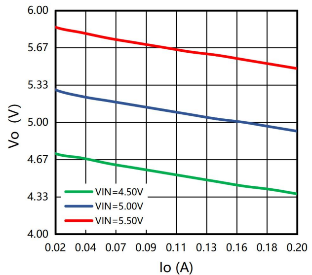
图 3: IO=0-200mA,VO 调整率曲线
