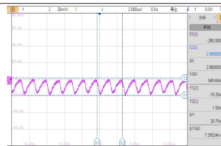
VIN=5V, 半载输出电压纹波波形
