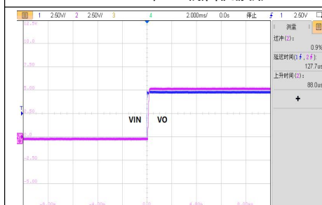
VIN=5V, 空载启机波形
