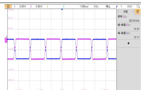
VIN=4.5V, 满载工作波形
