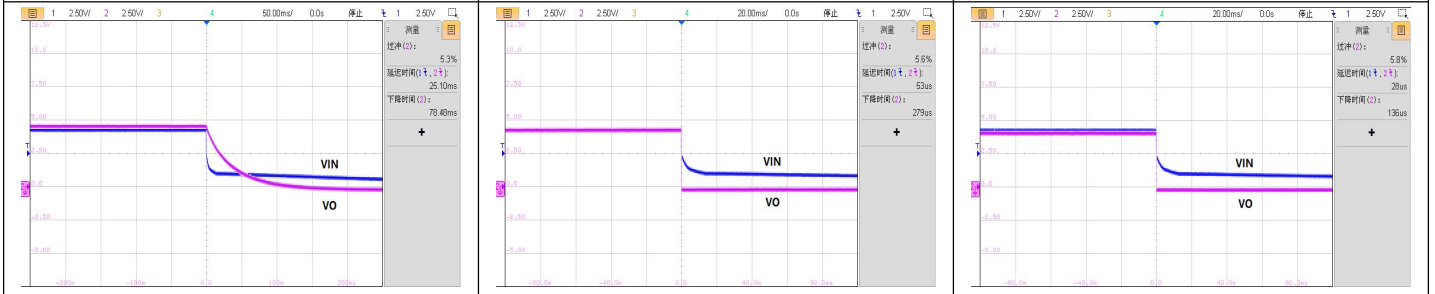
VIN=4.5V, 空载关机波形
