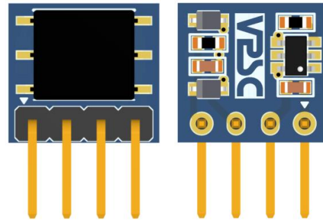
图 1: VPS8702B Demo 板(尺寸:11.16mm*10.32mm) 注: ▽ 为 1 脚
