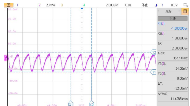
图 5: VIN=5V, IO=200mA,VO 输出电压纹波波形
