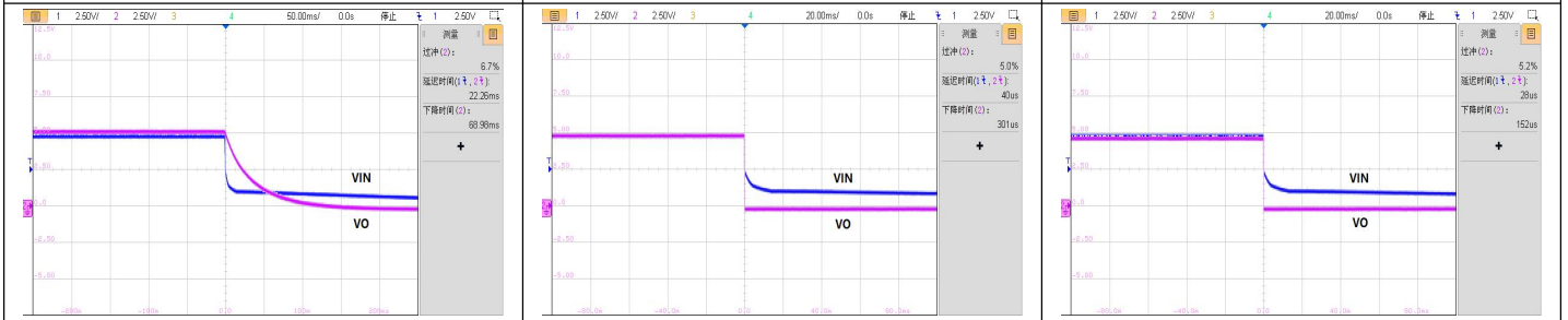
VIN=5.0V, 空载关机波形
