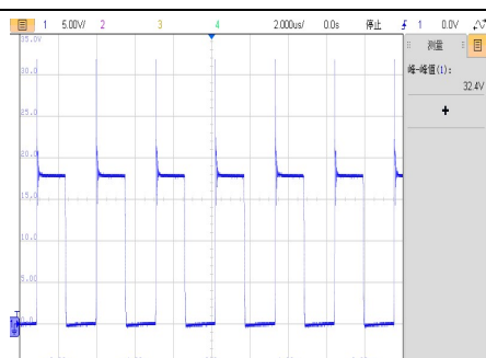
VIN=9V, 半载 VDS 波形
