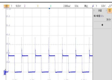
VIN=9V, 满载 VDS 波形
