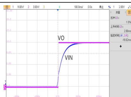
VIN=36V, 半载启机波形
