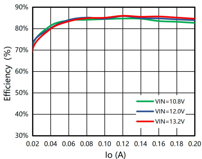
图 2: 满载效率 VS 输出电流
