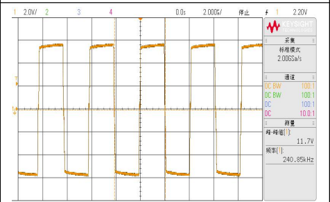
VIN=13.2V, 满载 VDS 波形
