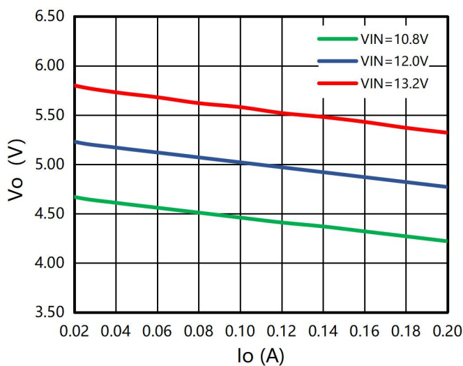
图 3: VO1 调整率曲线
