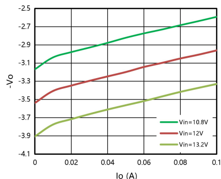
图 4: 负输出电压 VS 输出电流
