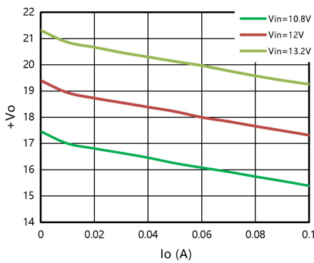
图 3: 正输出电压 VS 输出电流
