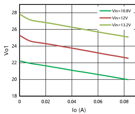
图 3: 输出电压1 VS 输出电流
