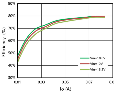
图 2: 效率 VS 输出电流
