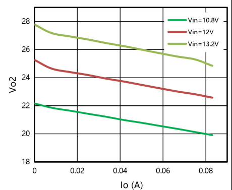
图 4: 输出电压2 VS 输出电流
