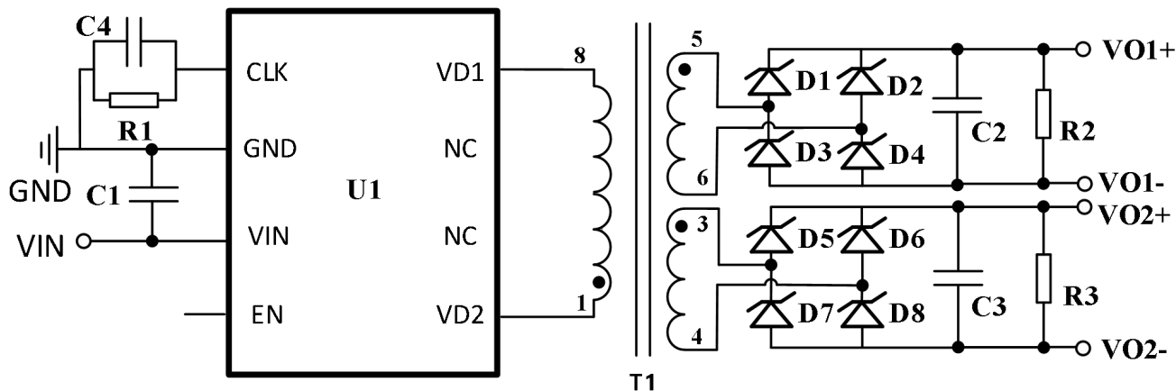
图 2：原理图
