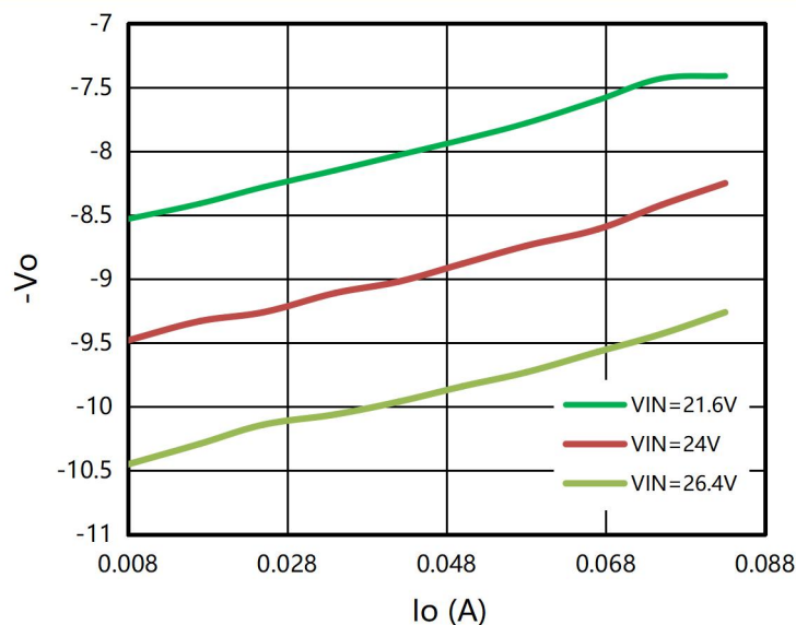
图 4: 负输出电压 VS 输出电流
