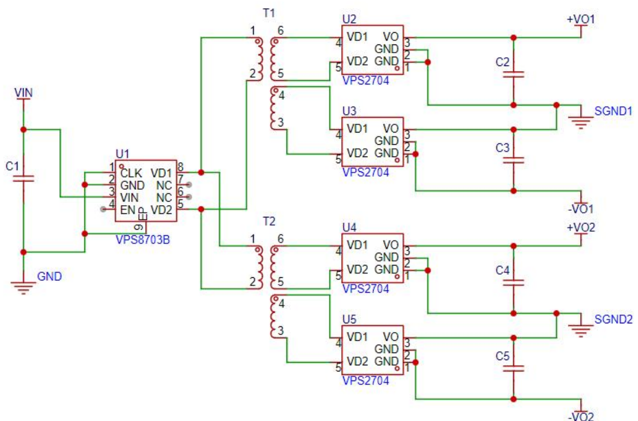
图 1: 原理图
