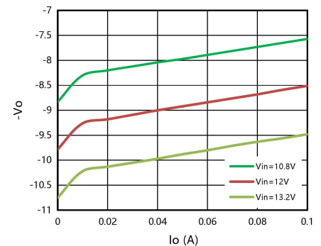
图 4: 负输出电压 VS 输出电流
