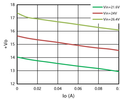
图 3: 正输出电压 VS 输出电流
