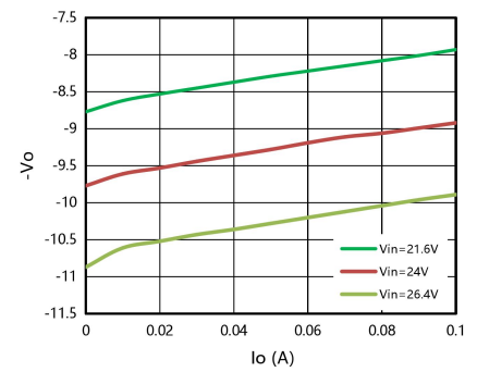
图 4: 负输出电压 VS 输出电流
