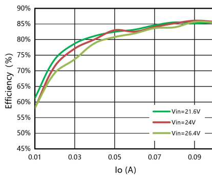
图 2: 效率 VS 输出电流
