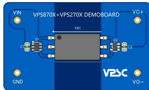
图 1: VPS8702 Demo 板(尺寸:50mm*30mm)
