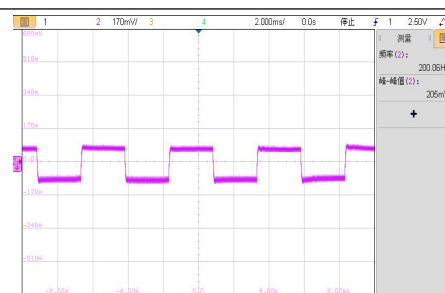
VIN=4.5V, 75%-50%-75%Io 动态波形
