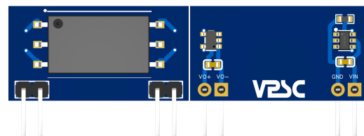
图 1: VPS8702 Demo 板(尺寸:27.4mm*14.5mm)
