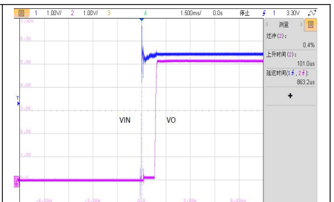
VIN=5.5V, 满载启机波形
