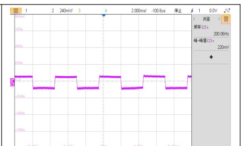
VIN=4.5V, 50%-25%-50%Io 动态波形
