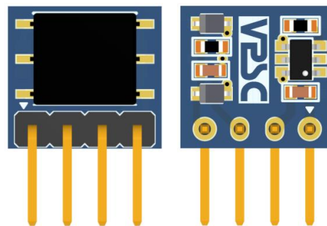
图 1: VPS8702 Demo 板(尺寸:11.16mm*10.32mm)
