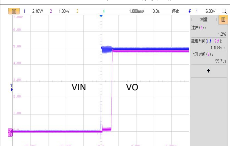
VIN=12.0V, 满载启机波形
