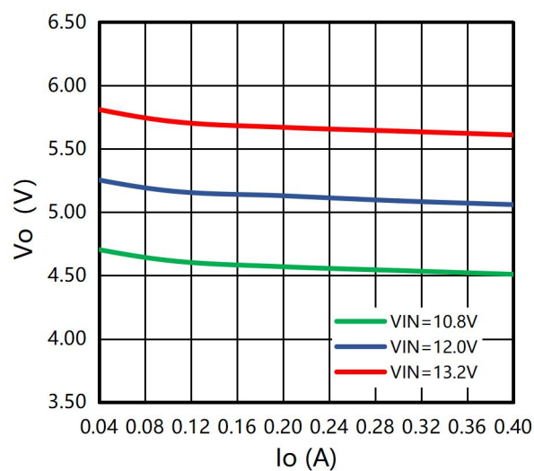
输出电压 VS 输出电流 (25°C)
