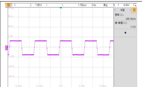
VIN=12.0V, 满载工作电压波形
