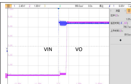
VIN=13.2V, 半载启机波形
