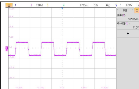
VIN=10.8V, 半载工作电压波形
