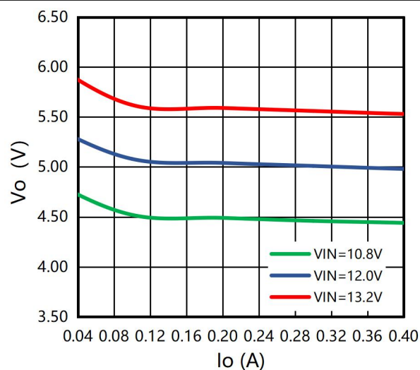
输出电压 VS 输出电流(-40°C)
