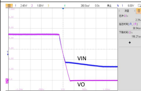
VIN=10.8V, 半载关机波形
