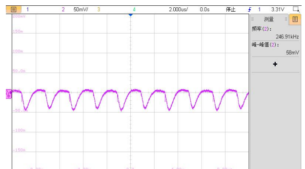
图 5: VIN=12.0V, 满载输出电压纹波波形
