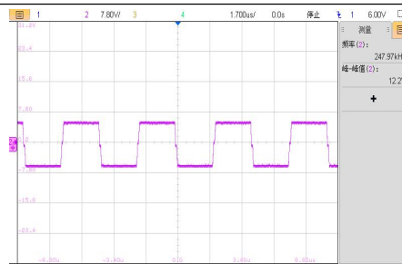
VIN=12.0V, 半载工作电压波形
