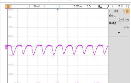
VIN=12.0V, 满载输出电压纹波波形
