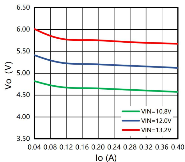
输出电压 VS 输出电流(85°C)
