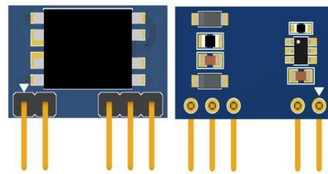
图 1: VPS8701B Demo 板 (19mm*12.0mm)
