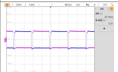
VIN=12.0V, 满载 VDS 波形
