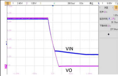
VIN=13.2V, 半载关机波形
