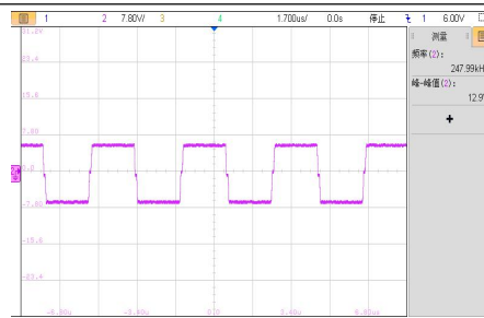
VIN=13.2V, 半载工作电压波形
