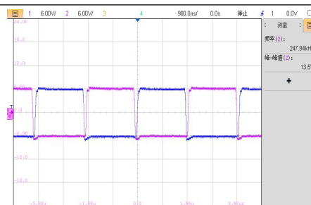
VIN=12.0V, 半载 VDS 波形
