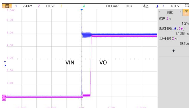
图 4: VIN=12.0V, 满载启机波形
