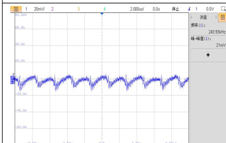
VIN=16.5V，轻载输出电压纹波波形
