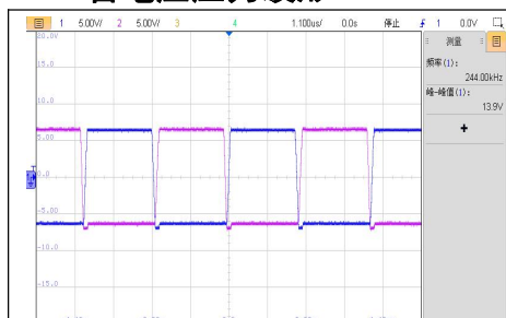
VIN=13.5V, 空载 VDS 波形
