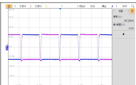
VIN=13.5V, 满载 VDS 波形
