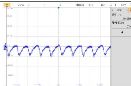
VIN=15V，半载输出电压纹波波形
