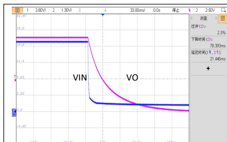
VIN=16.5V, 空载关机波形
