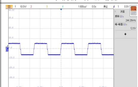
VIN=16.5V, 满载工作电压波形
