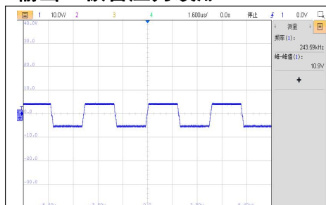
VIN=13.5V, 空载工作电压波形
