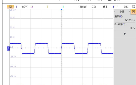
VIN=15V, 空载工作电压波形
