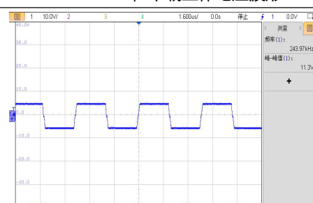
VIN=15V, 半载工作电压波形
