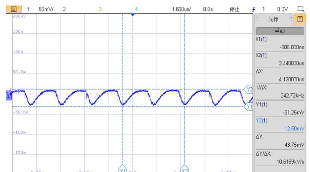
图 5: VIN=15V, 满载输出电压纹波波形
