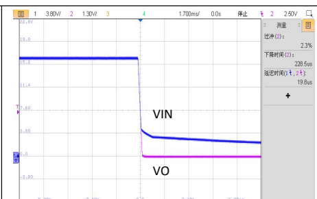
VIN=16.5V, 满载关机波形
