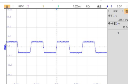
VIN=16.5V, 半载工作电压波形
