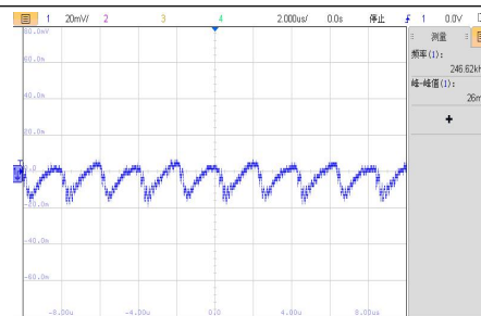
VIN=13.5V，半载输出电压纹波波形
