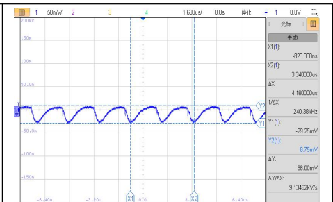
VIN=13.5V，满载输出电压纹波波形
