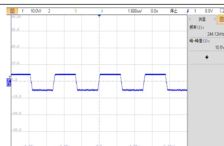
VIN=13.5V, 半载工作电压波形
