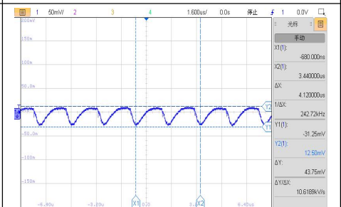
VIN=15V，满载输出电压纹波波形
