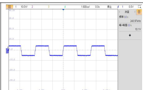
VIN=13.5V, 满载工作电压波形
