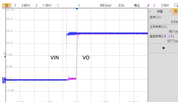
图 4: VIN=15V, 满载启机波形
