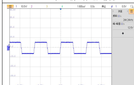
VIN=16.5V, 空载工作电压波形
