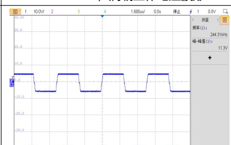
VIN=15V, 满载工作电压波形
