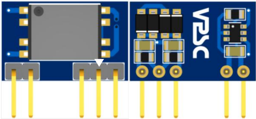
图 1: VPS8701B Demo 板 注: ▽为 1 脚
