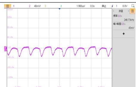
VIN=12V, 满载输出电压纹波波形
