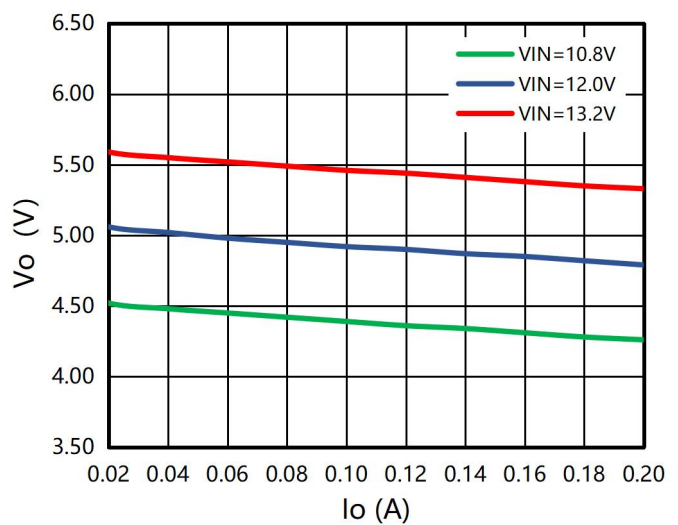
图 3: IO1/IO2=0-200mA,VO1 调整率曲线
