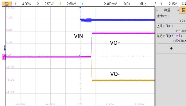
图 4: VIN=12V, IO1/IO2=200mA 启机波形
