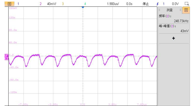
图 5: VIN=12V, IO1/IO2=200mA, VO1 输出电压纹波波形
