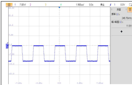
VIN=12V, 空载工作电压波形
