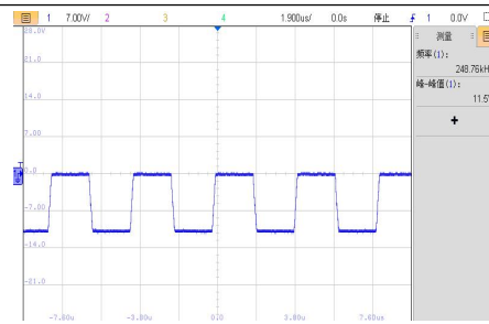
VIN=12V, 半载工作电压波形
