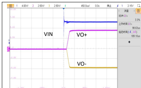
VIN=10.8V, 空载启机波形
