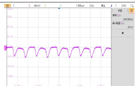
VIN=13.2V, 满载输出电压纹波波形
