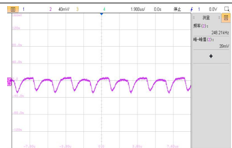
VIN=10.8V, 满载输出电压纹波波形
