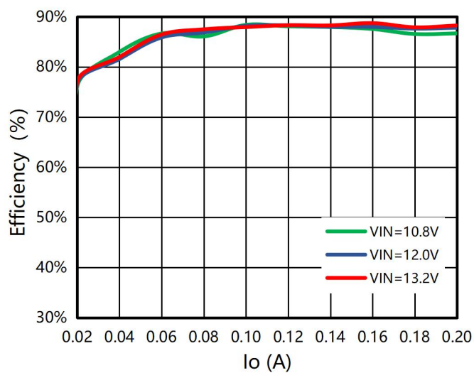
图 2: IO1/IO2=0-200mA,效率 VS 输出电流
