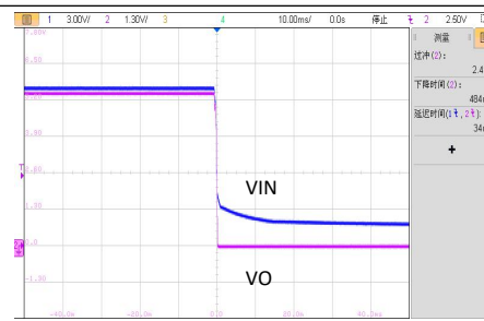
VIN=13.2V, 半载关机波形
