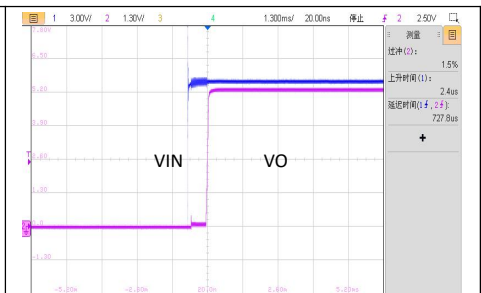
VIN=13.2V, 满载开机波形
