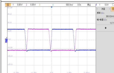
VIN=13.2V, 空载 VDS 波形
