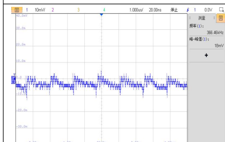
VIN=12V，轻载输出电压纹波波形
