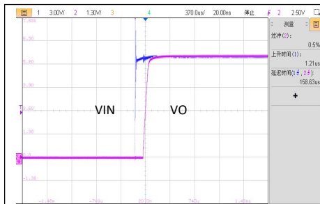
VIN=13.2V, 空载开机波形
