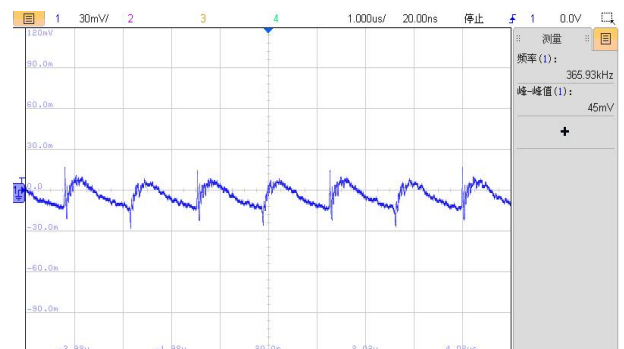
图 5: VIN=12V, 满载输出电压纹波波形
