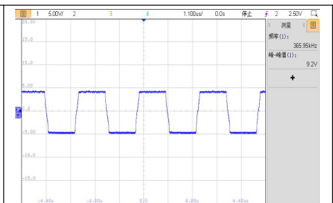
VIN=10.8V, 满载工作电压波形
