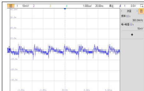
VIN=10.8V，轻载输出电压纹波波形
