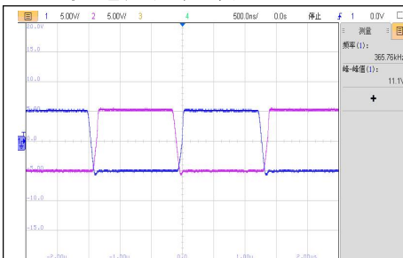
VIN=10.8V, 空载 VDS 波形
