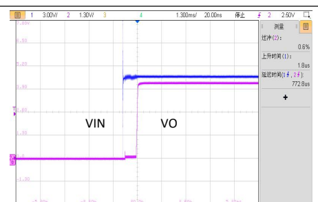
VIN=10.8V，满载启机波形
