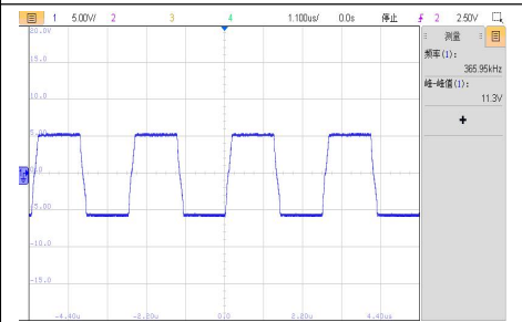
VIN=13.2V, 满载工作电压波形
