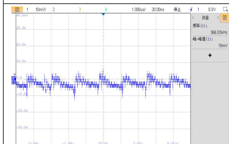
VIN=13.2V，轻载输出电压纹波波形
