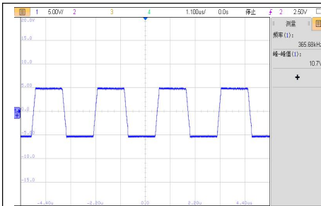
VIN=12V, 空载工作电压波形
