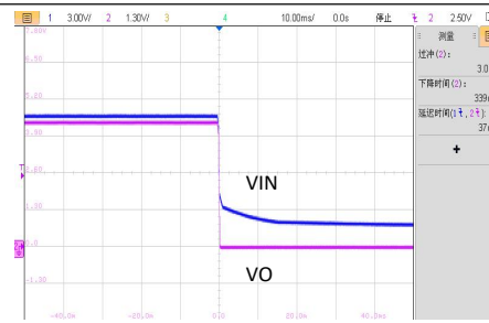
VIN=10.8V, 半载关机波形
