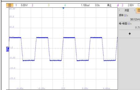
VIN=13.2V, 空载工作电压波形
