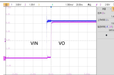
VIN=13.2V, 半载开机波形
