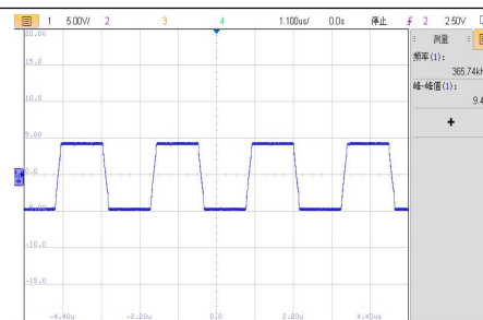
VIN=10.8V, 半载工作电压波形
