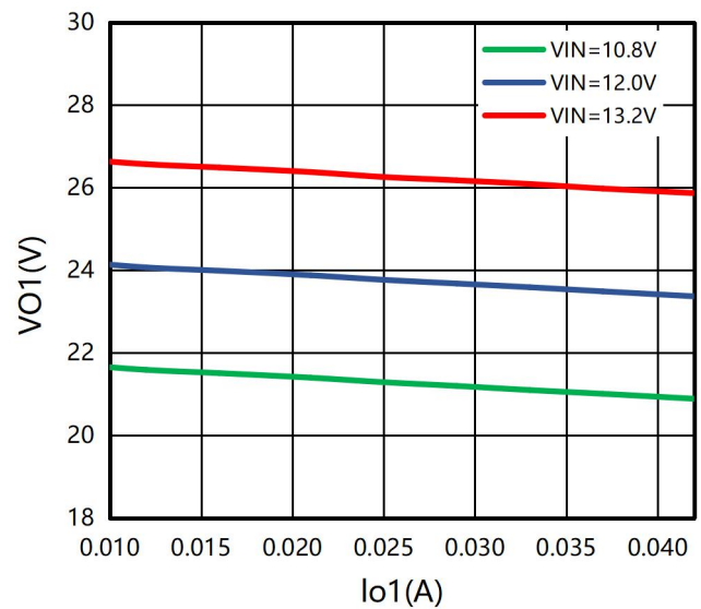
图 3: IO1/IO2=0-42mA,VO1 调整率曲线
