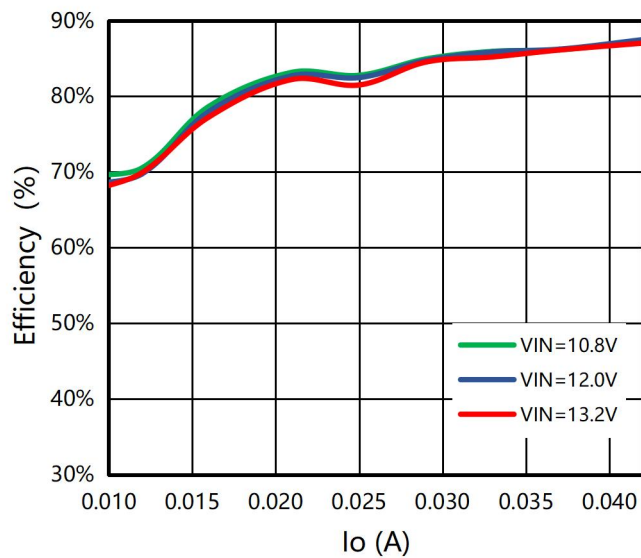
图 2: IO1/IO2=0-42mA,效率 VS 输出电流
