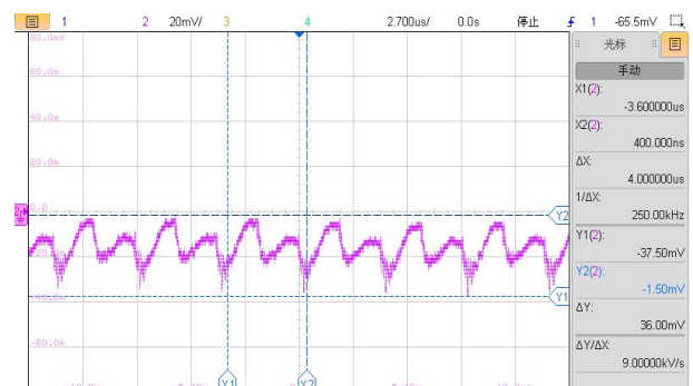
图 5: VIN=12V, IO1/IO2=42mA,VO1 输出电压纹波波形
