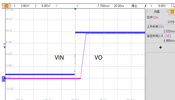
图 4: VIN=12V, IO1/IO2=42mA,VO1 启机波形
