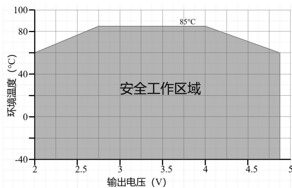
图 5 安全工作区域
