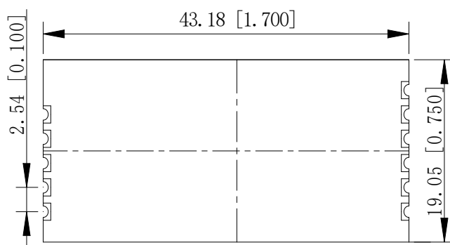
图 7 外观尺寸
