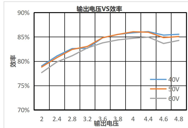
图 4 转换效率 VS 输出电压(25°C)
