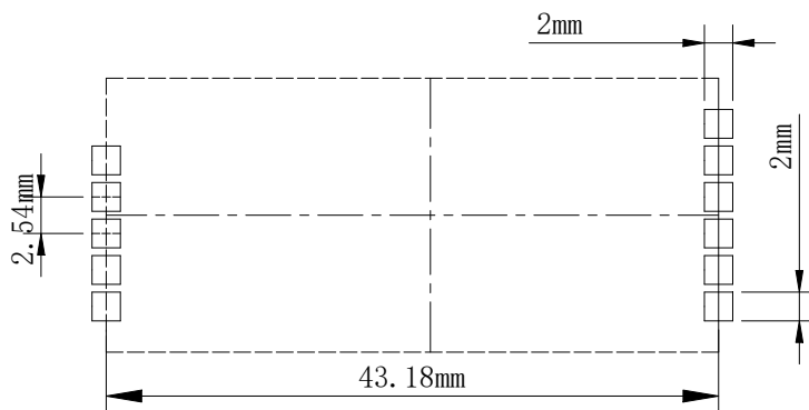
图 8 外观尺寸
