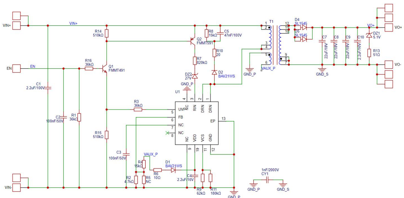
图 2 原理图
