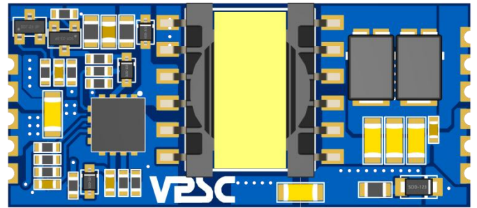
图 1 VPS2608 Demo 板 (尺寸:1700mil*750mil, 高度<10mm)
