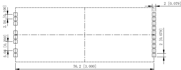
图 8 推荐封装
