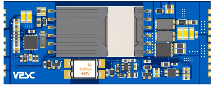
图 1 VPS2606 Demo 板 (布板尺寸:72mm*28mm, 高度<10mm)
