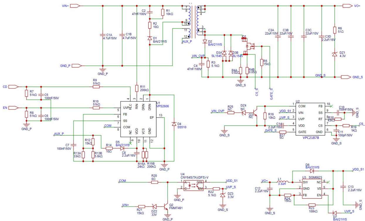
图 2 原理图
