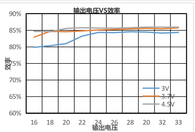
图 4 反向工作，转换效率 VS 输出电压(25°C)
