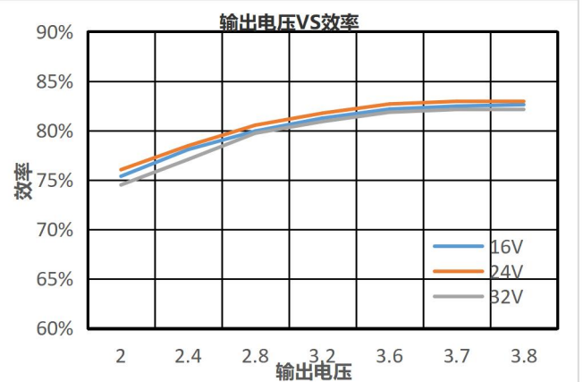
图 4 正向工作，转换效率 VS 输出电压(25°C)
