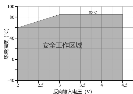
图 5 反向工作安全工作区域
