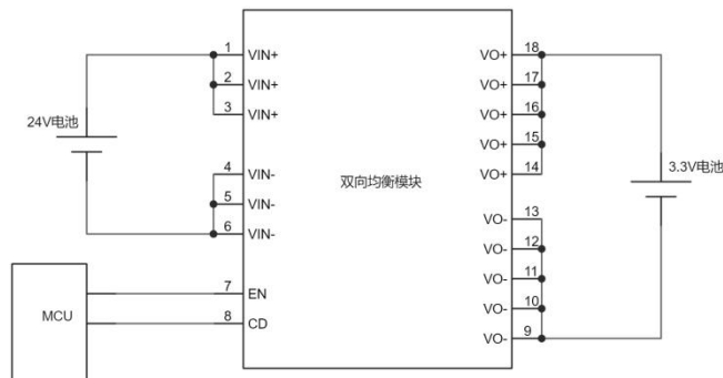
图 6 参考设计
