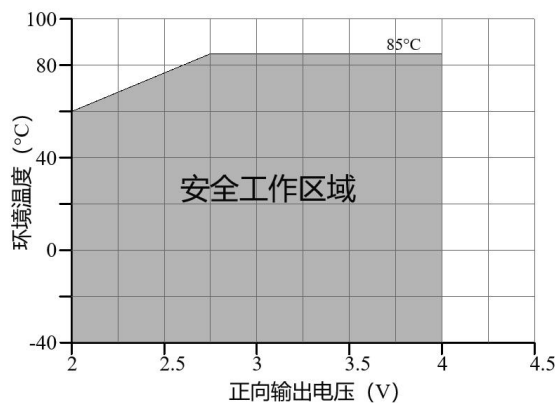
图 5 正向工作安全工作区域
