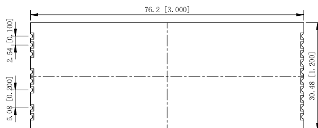
图 7 外观尺寸
