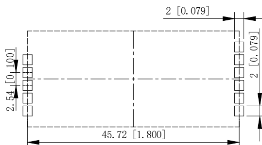
图 8 推荐封装
