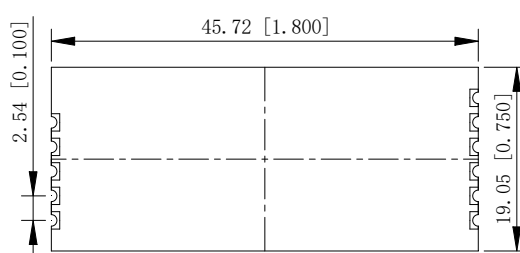
图 7 外观尺寸
