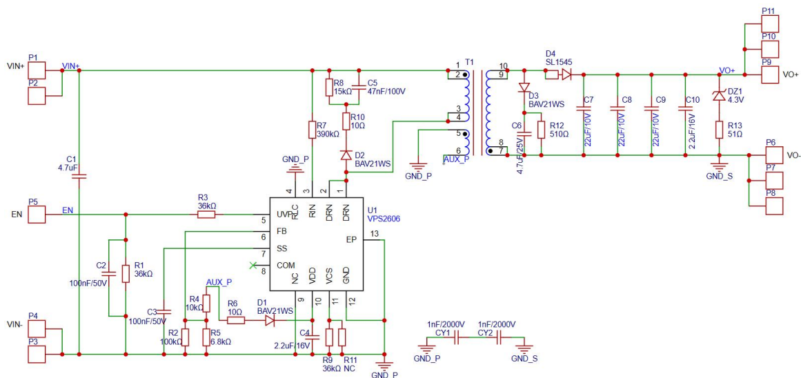
图 2 原理图
