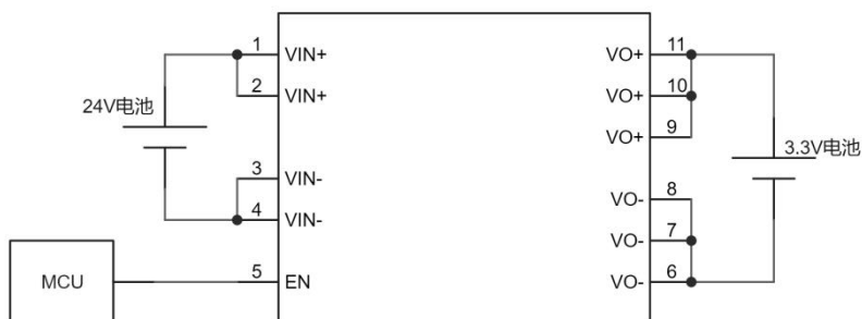
图 6 参考设计
