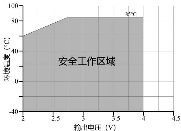
图 5 安全工作区域
