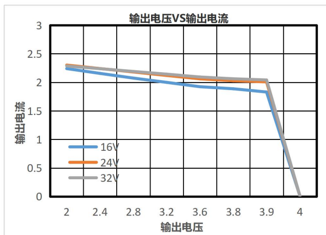
图 3 输入电压 vs 输出电流(25°C)
