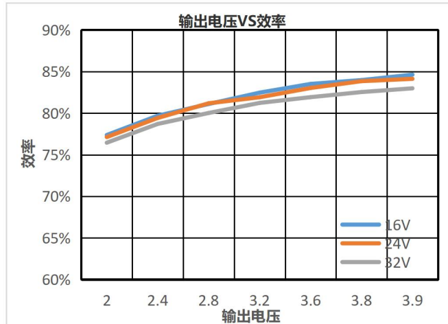
图 4 转换效率 VS 输出电压(25°C)
