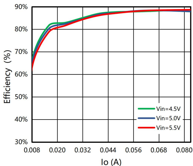
图 2: 效率 VS 输出电流曲线(输出满载)
