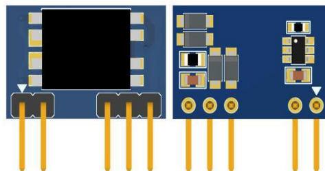
图 1: VPS8504B Demo 板(尺寸:19mm*12mm)
