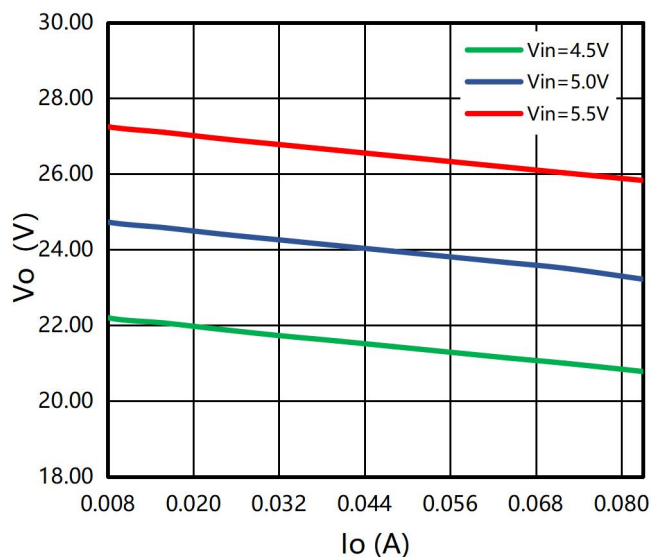
图 3: 输出电压 VS 输出电流曲线
