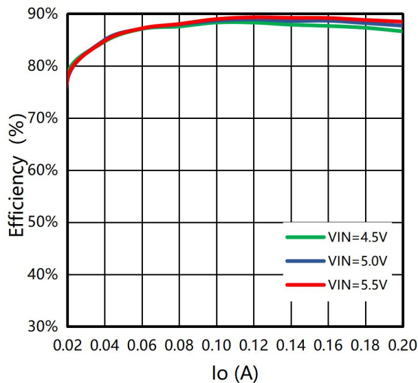
图 2: IO1/IO2=0-200mA,效率 VS 输出电流
