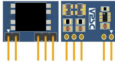
图 1: VPS8504B Demo 板
