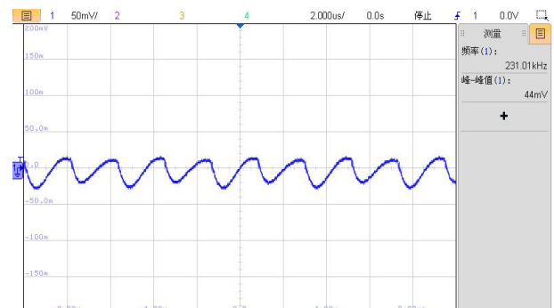
图 5: VIN=5V, IO1/IO2=200mA,VO1 输出电压纹波波形
