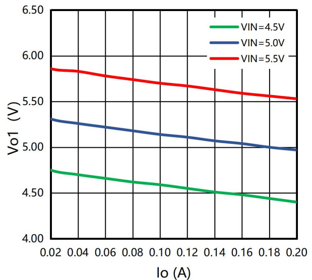
图 3: IO1/IO2=0-200mA,VO1 调整率曲线
