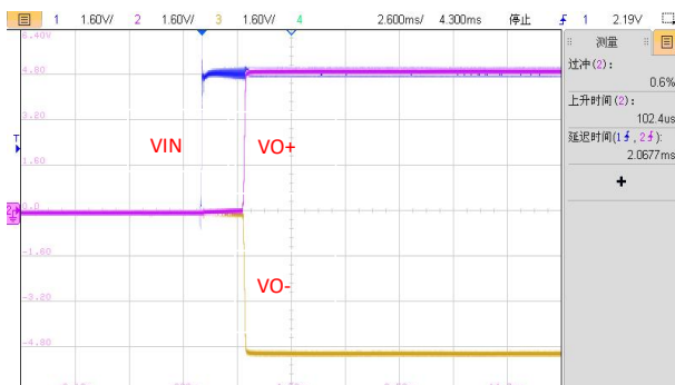
图 4: VIN=5V, IO1/IO2=200mA,VO1 开机波形
