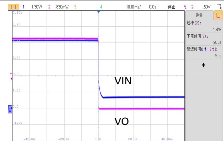
VIN=5.5V, 满载关机波形
