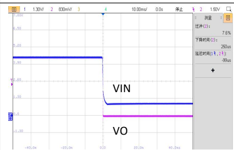
VIN=4.5V, 满载关机波形
