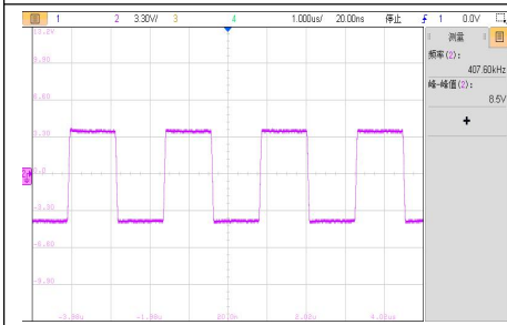
VIN=5.5V, 空载工作电压波形
