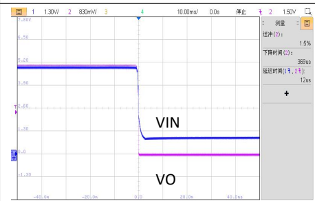
VIN=5.0V, 满载关机波形
