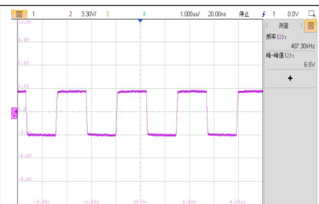
VIN=4.5V, 满载工作电压波形
