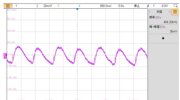
图 5: VIN=3.3V，满载输出电压纹波波形
