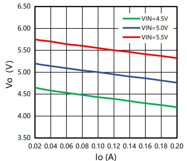
图 3: 输出电压 VS 输出电流
