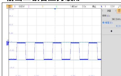
VIN=4.5V, 空载工作电压波形
