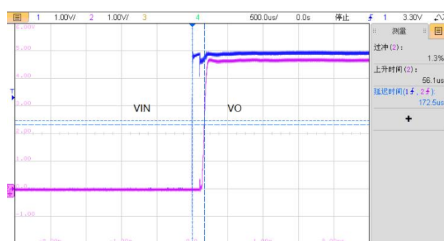
图 4: VIN=5V, 满载启机波形
