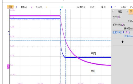
VIN=5.0V, 空载关机波形
