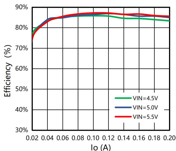
图 2: 效率 VS 输出电流(输出满载)
