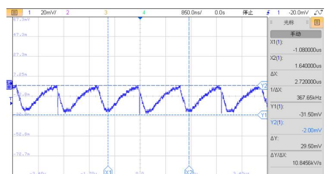
图 5: VIN=5V, 满载输出电压纹波波形
