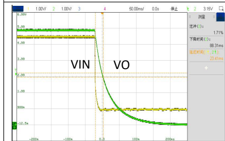
VIN=5.5V, 空载关机波形
