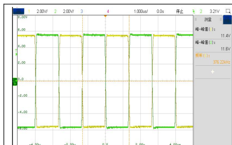
VIN=5V, 空载工作波形
