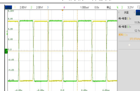
VIN=5.5V, 满载工作波形
