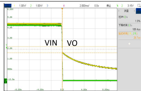
VIN=5.5V, 满载关机波形
