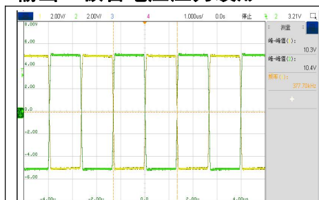
VIN=4.5V, 空载工作波形
