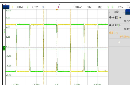
VIN=4.5V, 半载工作波形
