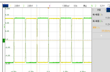
VIN=5V, 半载工作波形
