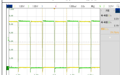
VIN=5.5V, 空载 VDS 波形
