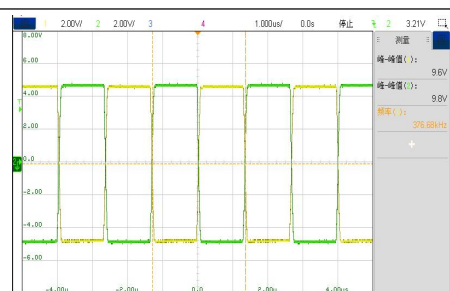
VIN=4.5V, 满载工作波形
