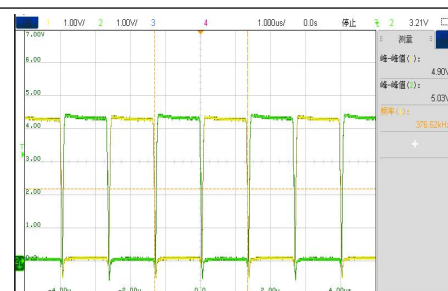
VIN=4.5V, 满载 VDS 波形
