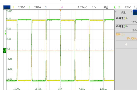
VIN=5.5V, 半载工作波形
