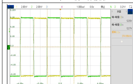
VIN=5.5V, 空载工作波形
