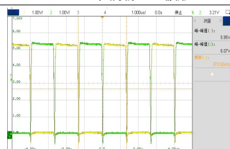
VIN=5.5V, 满载 VDS 波形
