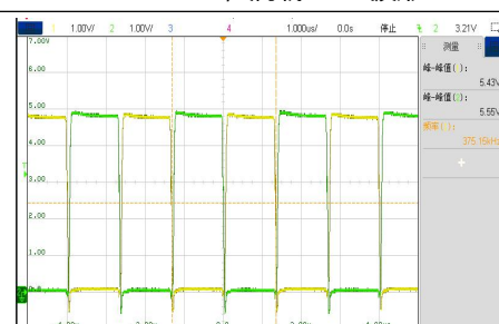
VIN=5V, 满载 VDS 波形
