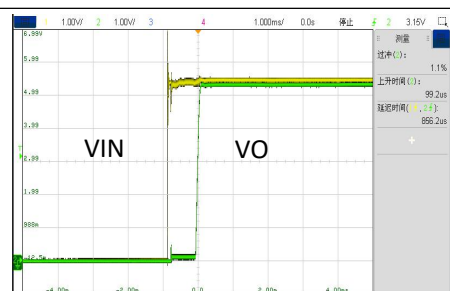
VIN=5.5V, 满载启机波形
