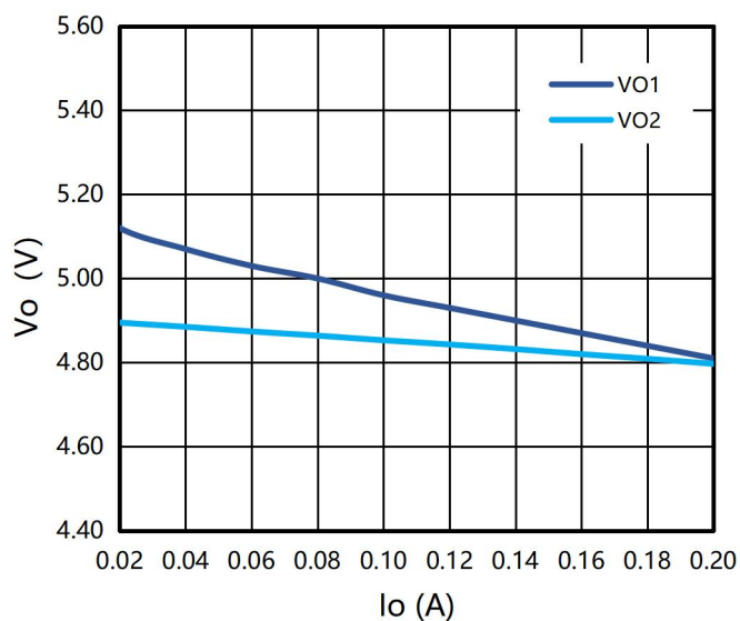
图 3: VO1/VO2 调整率 (IO2 满载)
