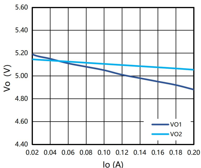
图 2: VO1/VO2 调整率 (IO2 半载)
