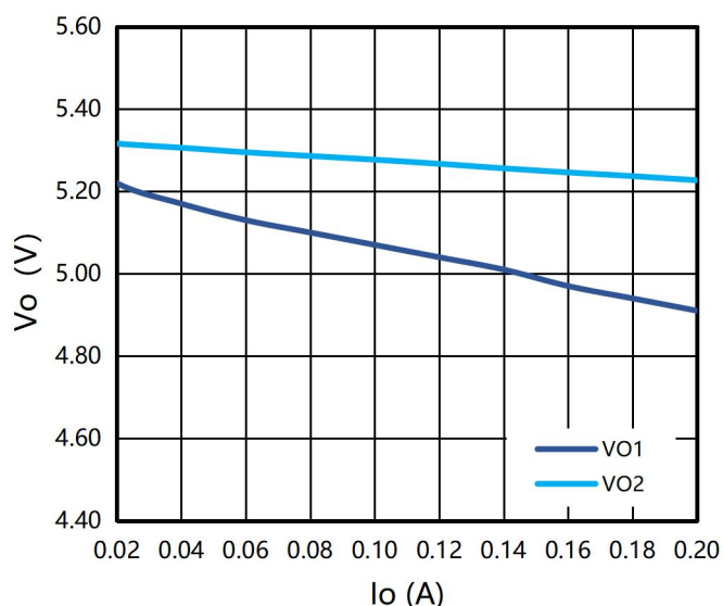
图 1: VO1/VO2 调整率 (IO2 空载)
