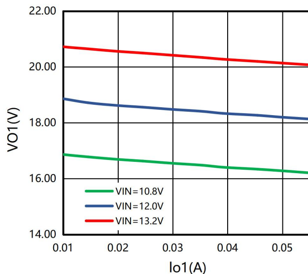
图 3: IO1=0-56mA,VO1 调整率曲线
