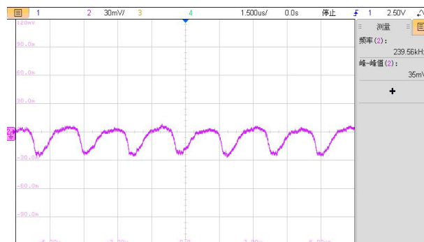
图 6: VIN=12V, IO1=56mA,VO1 输出电压纹波波形
