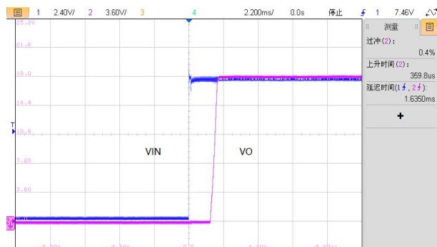
图 5: VIN=12V, IO1=56mA,VO1 启机波形
