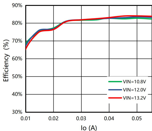
图 2: IO1=0-56mA,效率 VS 输出电流
