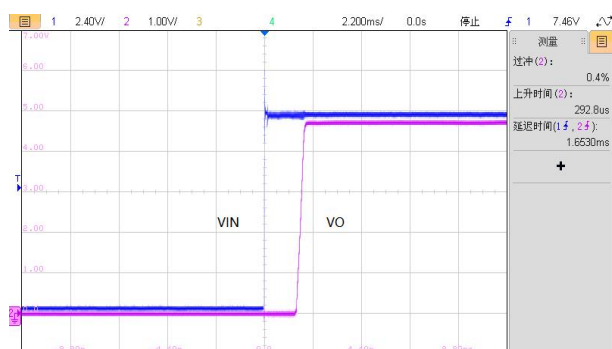
图 5: VIN=12V, IO2=200mA,VO1 启机波形
