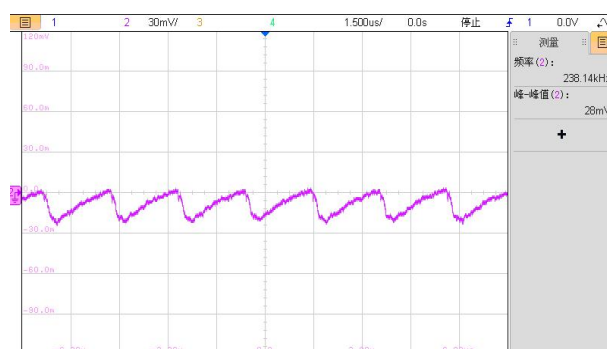
图 6: VIN=12V, IO2=200mA,VO1 输出电压纹波波形
