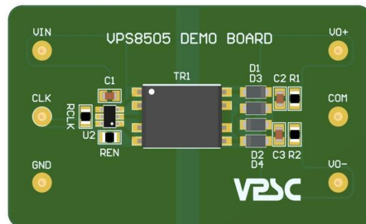
图 1: VPS8505 Demo 板(尺寸:50mm*30mm)
