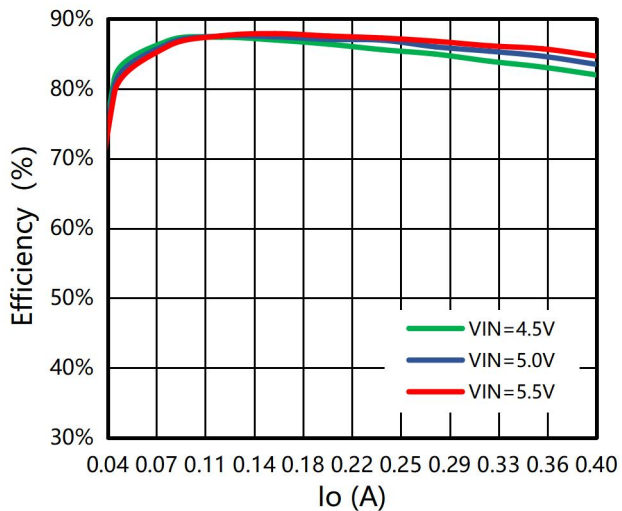
效率 VS 输出电流(85°C)
