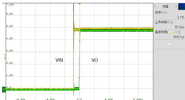
图 4: VIN=5V, 满载启机波形
