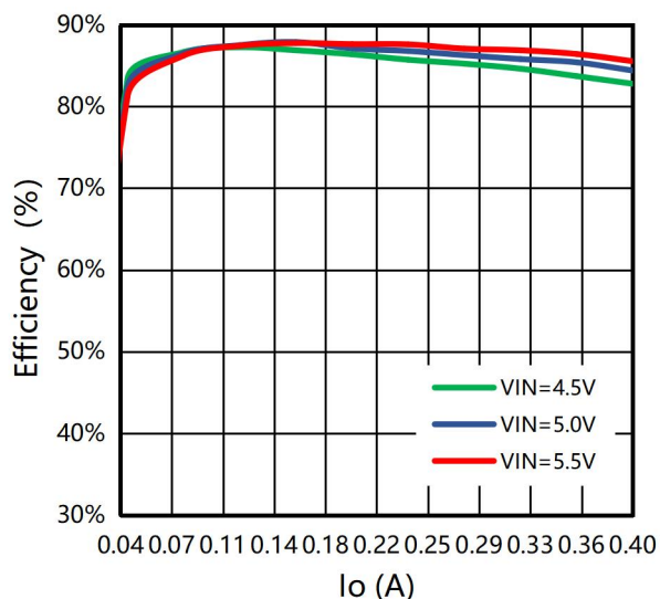
图 2: 效率 VS 输出电流(输出满载)
