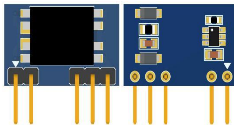
图 1: VPS8504B Demo 板(尺寸:14.68mm*12.44mm) 注: ▽ 为 1 脚
