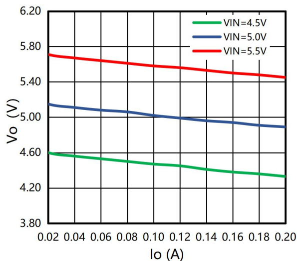
输出电压 VS 输出电流(输出满载@-40°C)
