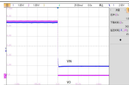
VIN=5.5V，半载关机波形
