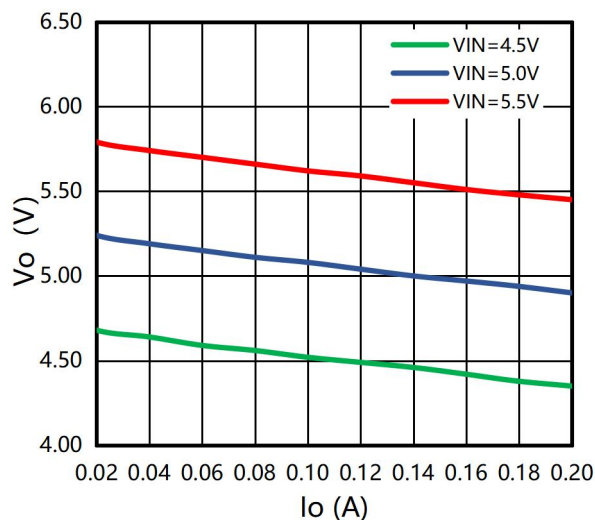
输出电压 VS 输出电流(输出满载@25°C)
