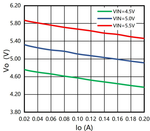
输出电压 VS 输出电流(输出满载@85°C)
