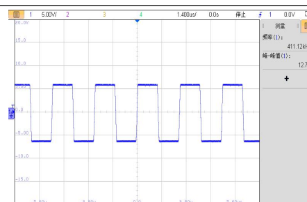
VIN=5.5V, 半载工作电压波形
