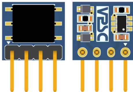
图 1: VPS8504B Demo 板(尺寸:11.16mm*10.32mm) 注: ▽ 为 1 脚
