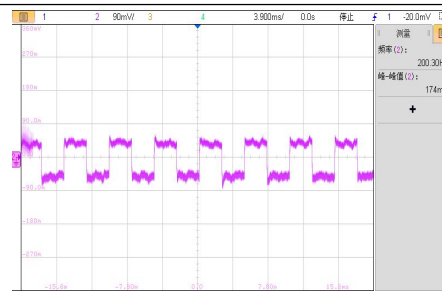
VIN=5.0V, 75%-50%-75%Io 动态波形
