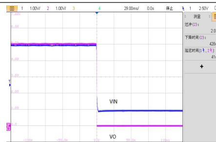
VIN=5.0V，半载关机波形
