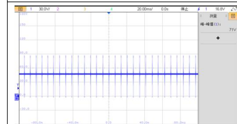
VIN=48V，空载 VDS 波形
