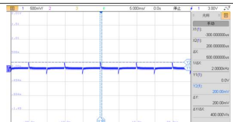
VIN=60V，50%-25%-50%Io 动态波形
