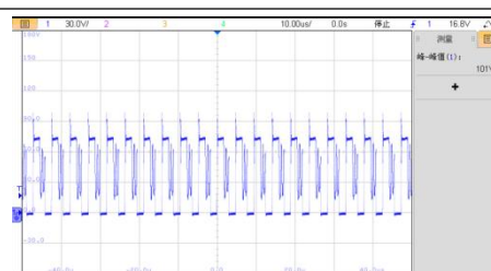
VIN=37V，半载 VDS 波形
