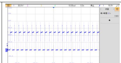
VIN=37V，满载 VDS 波形
