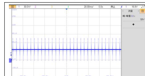
VIN=37V，空载 VDS 波形
