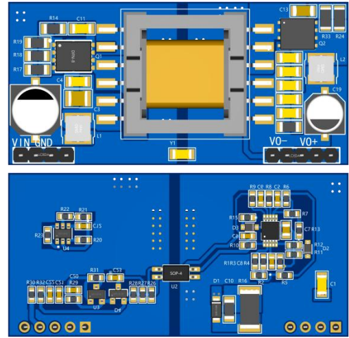
图 1: VPC2188B Demo 板(尺寸:56.9mm*27mm)
