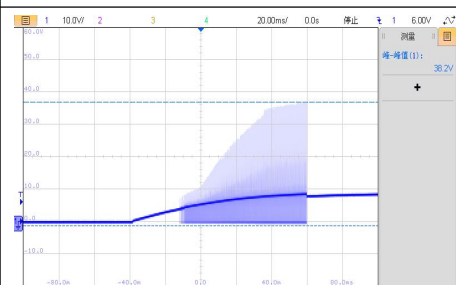
VIN=9V, 短路启机 VDS 波形
