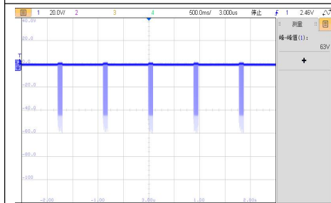
VIN=60V, D4 短路保护电压波形
