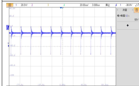
VIN=60V, D4 空载工作电压波形
