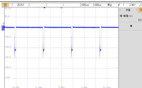
VIN=60V, D4 短路保护电压展开波形
