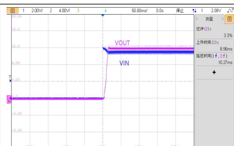
VIN=6V, 满载启机波形
