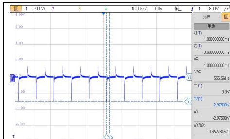
VIN=6V, 100%-10%-100%lo 动态波形
