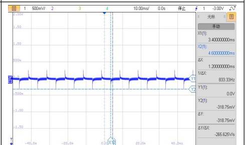
VIN=48V, 50%-25%-50%Io 动态波形
