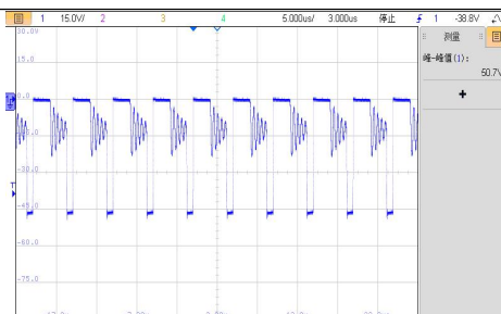
VIN=48V, D4 半载工作电压波形
