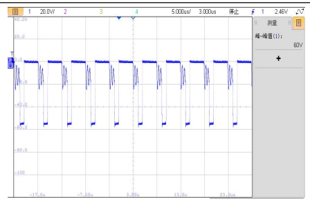
VIN=60V, D4 满载工作电压波形
