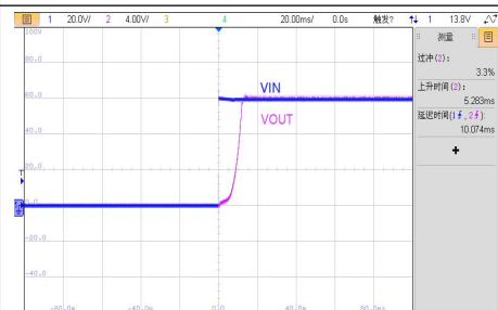
VIN=60V, 满载启机波形
