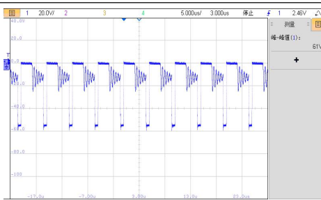
VIN=60V, D4 半载工作电压波形
