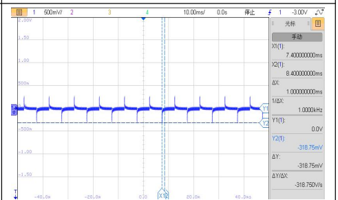
VIN=60V, 50%-25%-50%Io 动态波形
