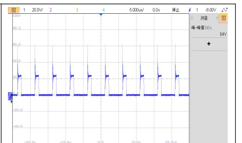
VIN=6V, 满载 VDS 波形
