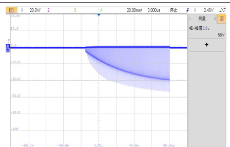
VIN=60V, D4 短路保护启机电压波形
