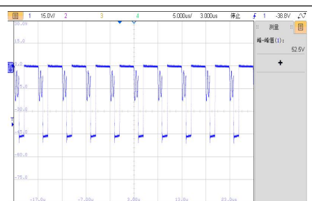
VIN=48V, D4 满载工作电压波形
