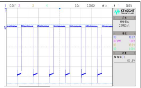
VIN=72V, D4 满载工作电压波形
