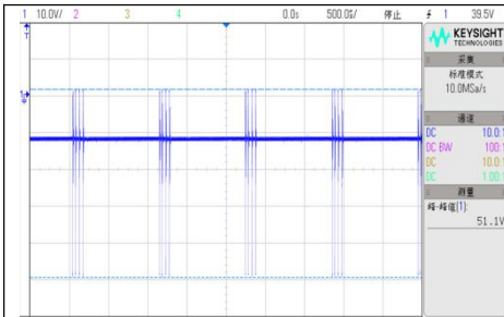
VIN=72V, D4 空载工作电压波形
