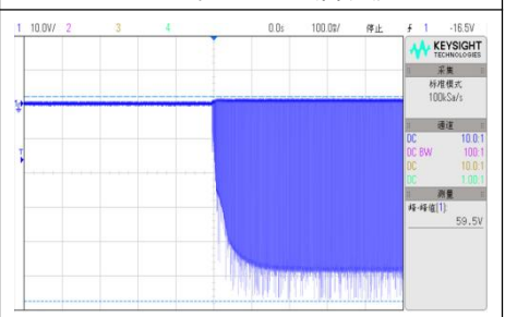
VIN=72V, D4 满载启机波形
