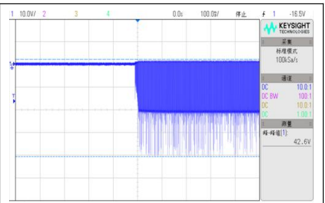
VIN=18V, D4 满载启机波形
