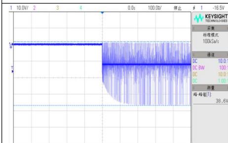
VIN=48V, D4 空载启机波形
