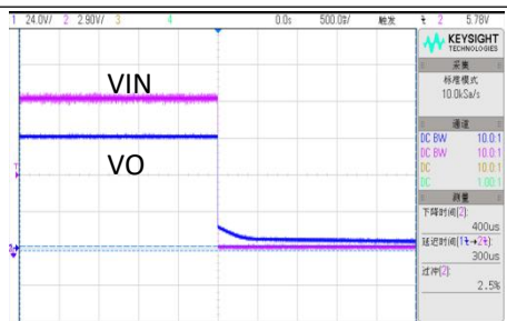
VIN=72V, 满载关机波形
