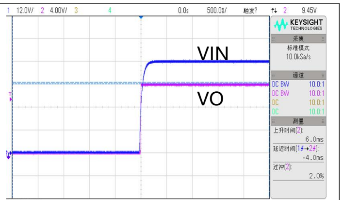
图 6: VIN=48V, 满载启机波形
