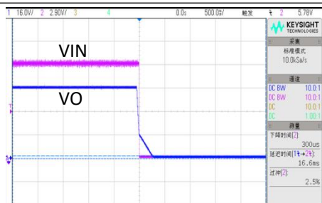
VIN=48V, 满载关机波形
