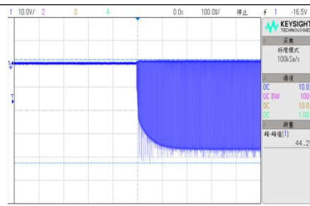
VIN=48V, D4 半载启机波形
