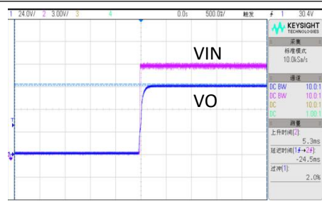
VIN=72V, 满载启机波形
