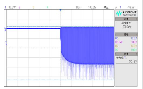
VIN=48V, D4 满载启机波形
