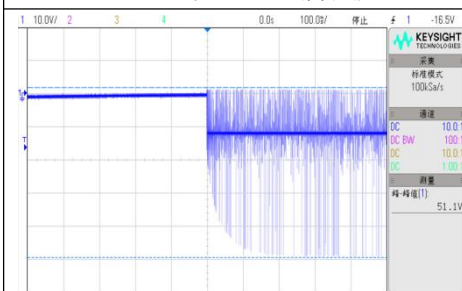
VIN=72V, D4 空载启机波形
