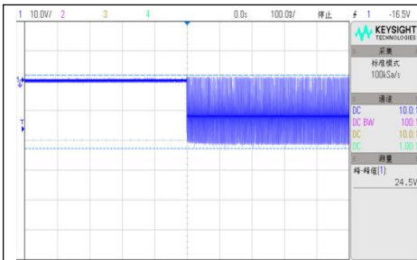
VIN=18V, D4 空载启机波形
