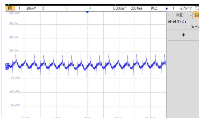
图 5: VIN=48V, 满载输出电压纹波波形
