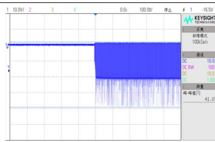
VIN=18V, D4 半载启机波形
