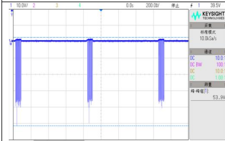
VIN=72V, D4 短路保护工作电压波形
