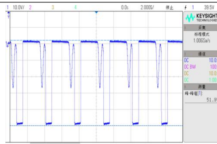
VIN=72V, D4 半载工作电压波形
