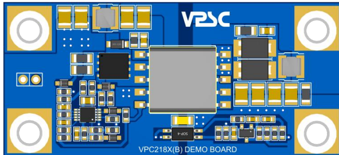
图 1: VPC2187B Demo 板(尺寸:67.5mm*30.7m)
