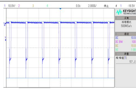
VIN=72V, D4 短路保护工作电压展开波形
