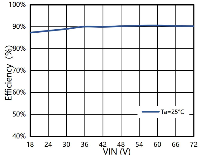
图 4: 效率 VS 输入电压 (输出满载@25°C)
