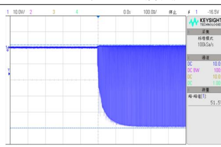
VIN=72V, D4 半载启机波形
