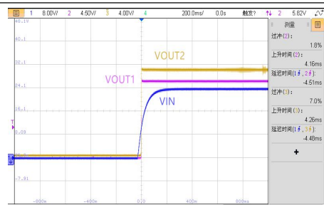
VIN=24V, 半载启机波形
