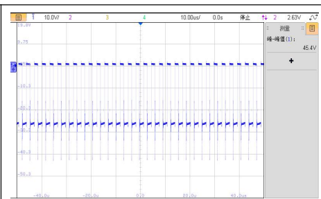
VIN=9V, 满载工作电压波形
