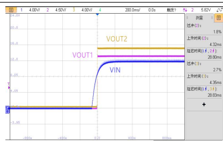
VIN=12V, 半载启机波形
