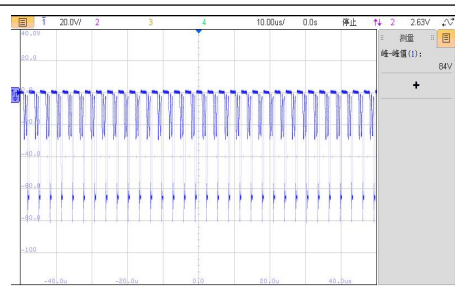
VIN=36V, 半载工作电压波形
