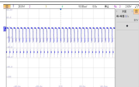
VIN=24V, D4 半载工作电压波形
