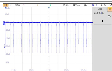
VIN=36V, 满载短路电压展开波形
