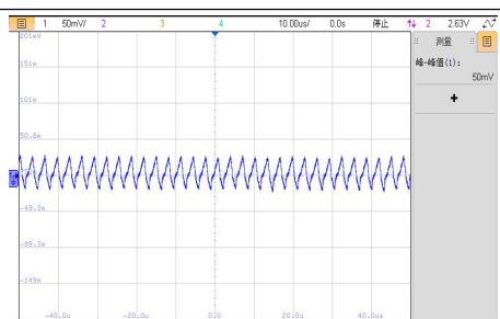
VIN=24V, 满载输出电压纹波波形
