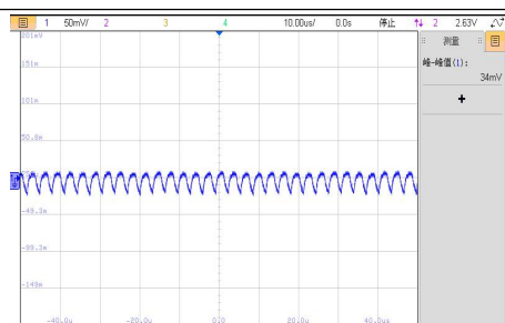
VIN=24V, 半载输出电压纹波波形
