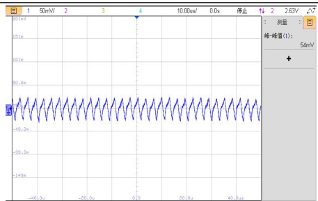
VIN=36V, 满载输出电压纹波波形
