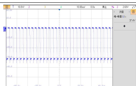
VIN=12V, 半载工作电压波形
