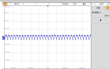
VIN=36V, 半载输出电压纹波波形
